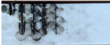
Rys. 5. Polipropylen (a-c) i polipropylen z talkiem (d-f) przecięty z prędkościami (od lewej): 1, 2, 3, 4, 6, 8, 10, 15 i 20 mm/s przy mocy lasera ok. 70W (99%)
