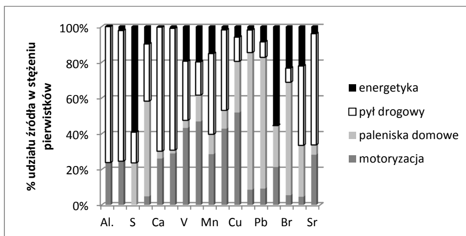
Rys. 4. Profile źródeł emisji oraz udziały ich w stężeniach pierwiastków rejestrowanych w receptorze
