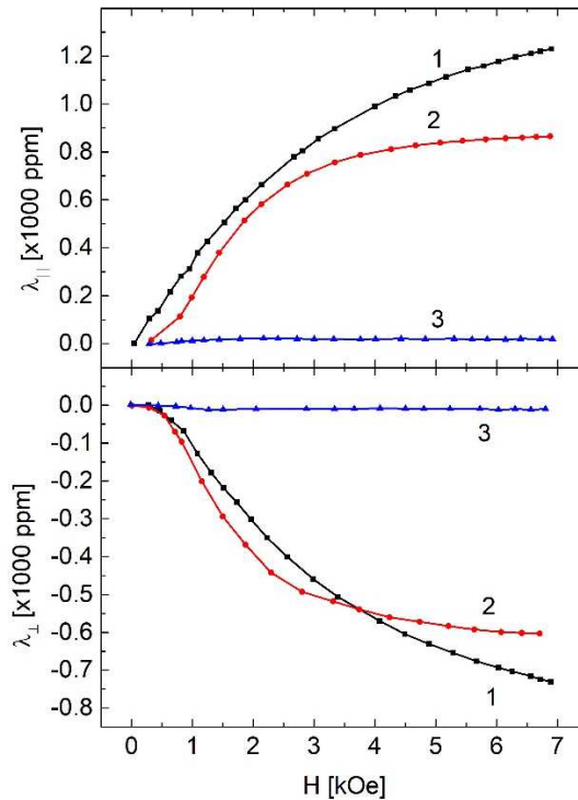
Rys. 8. Zależność magnetostrykcji podłużnej \lambda_{\parallel} i poprzecznej \lambda_{\perp} od natężenia H zewnętrznego pola magnetycznego dla związków: 1 – TbFe_2 , 2 – Tb_{0.27} Dy_{0.73} Fe_2 i 3 – YFe_2 .
