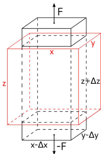
Rys. 1. Naprężenie i odkształcenie prostokątnej próbki jako wynik działającej siły F ; czerwony kontur – przed zadziałaniem siły F , czarny kontur – wynik działającej siły F
