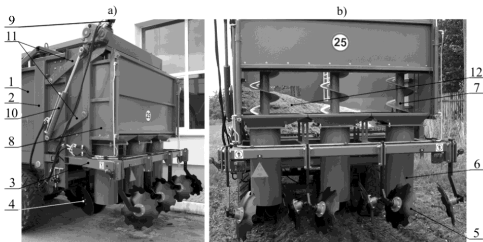
Rys. 3. Prototyp urządzenia do iniekcijnego dawkowania do gleby sypkich nawozów organicznych i mineralnych firmy R&D Centre Inventor Lublin sp. z o.o. – widok z boku (a) oraz z tyłu (b): 1 – rozrzutnik nawozów, 2 – rama nośna, 3 – belka, 4 – krój tarczowy, 5 – obsypnik talerzowy, 6 – cylindryczna obudowa ślimaka, 7 – podajnik ślimakowy, 8 – komora zasypowa, 9 – silnik hydrauliczny, 10 – siłownik hydrauliczny, 11 – ramiona, 12 – nawóz
